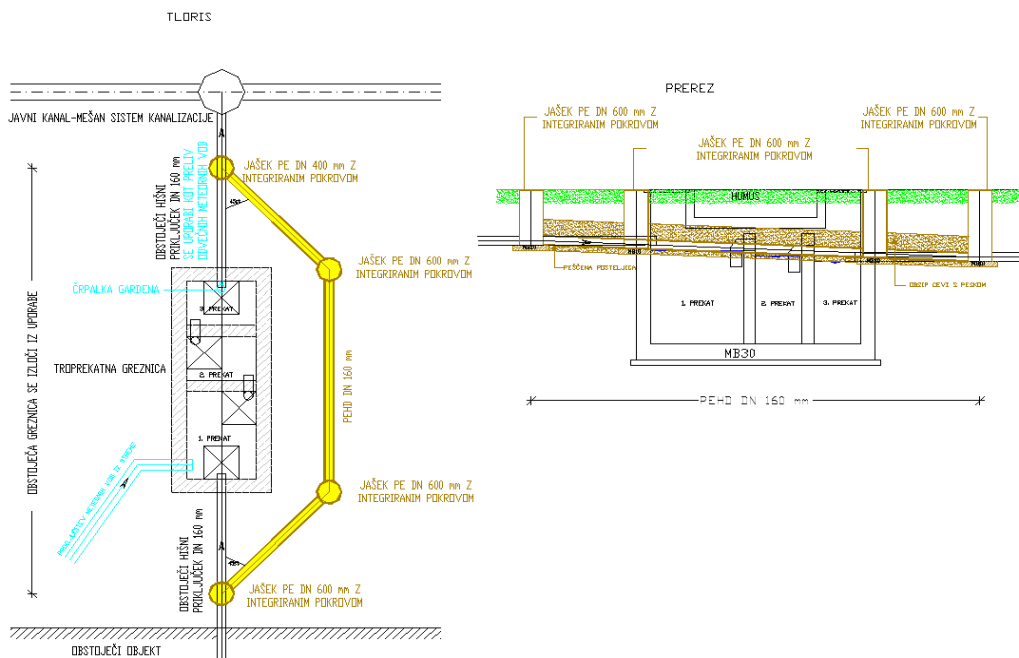
Opustitev greznice – povezava okrog greznice
