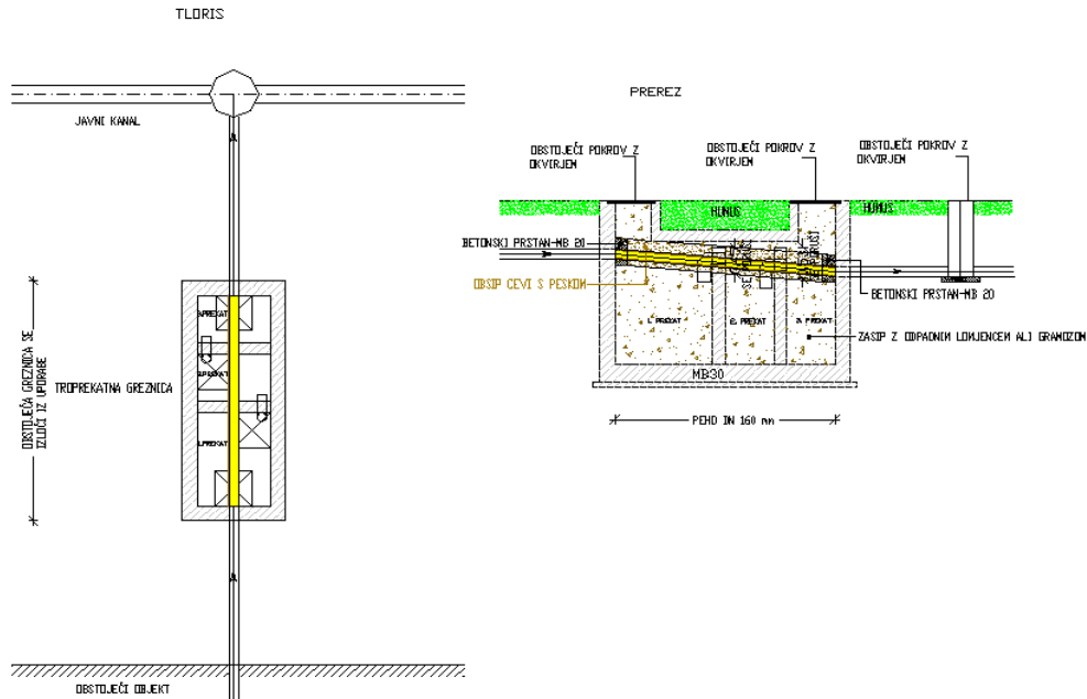
Opustitev greznice – povezava skozi greznico
